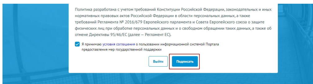
Рисунок 7. Кнопка «Подписать»
