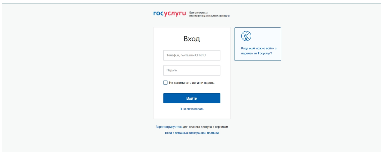
Рисунок 4. Окно авторизации
