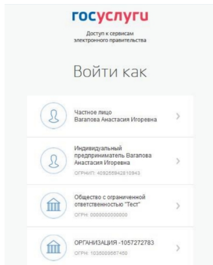
Рисунок 8. Выбор роли
