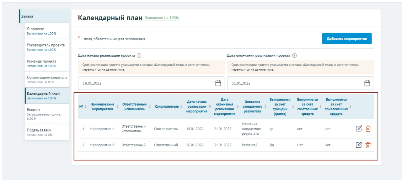
Рисунок 36. Таблица мероприятий
