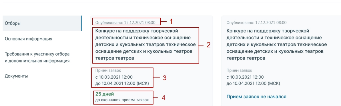
Рисунок 22. Карточка отбора
