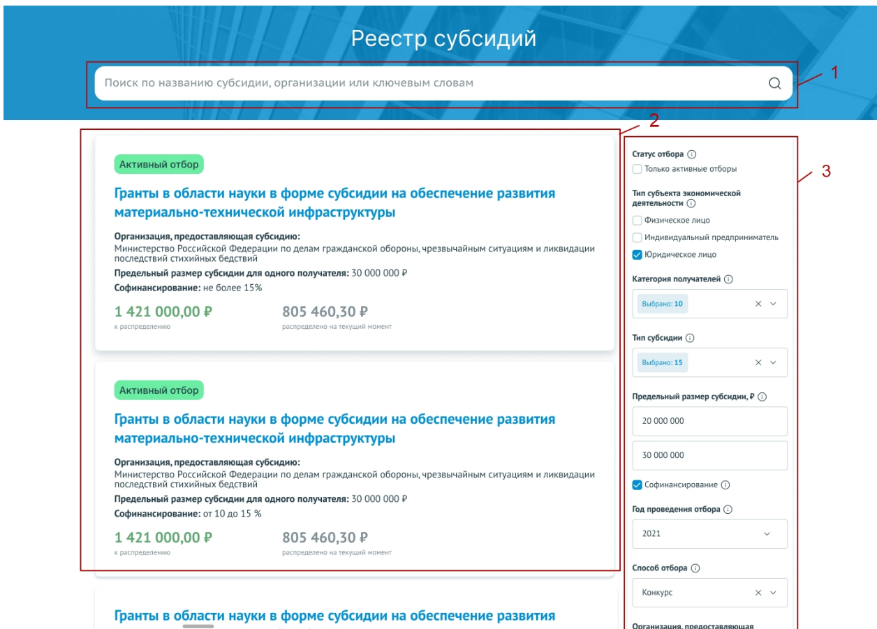
Рисунок 18. «Реестр субсидий»
