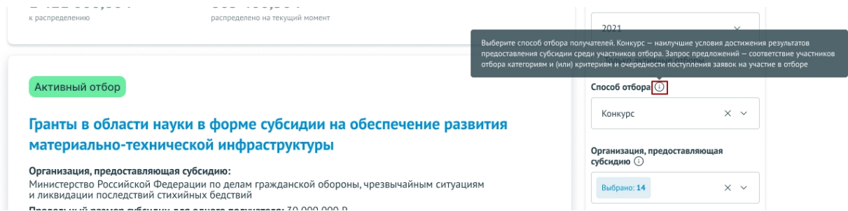
Рисунок 19. Подсказка фильтра
