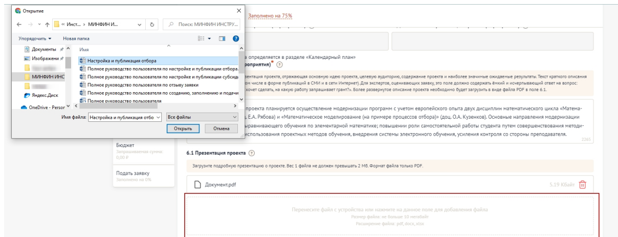
Рисунок 29. Диспетчер загрузки
