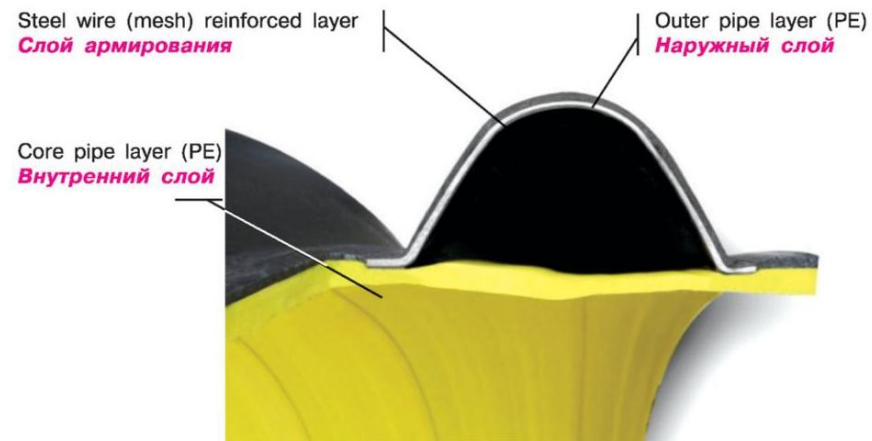
Разрез канализационной безнапорной полиэтиленовой армированной трубы
