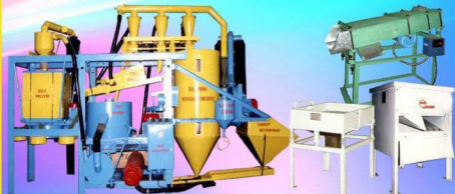
Универсальные мельничные комплексы Мукопросеиватели ручные МПВ120 Мукопросеиватели электрические Челябинская обл. ФКУ ИК-10, Саратовская обл. ФКУ ИК-2, Пензенская обл. ФКУ ИК-1, Владимирская обл. ФКУ ИК-7
